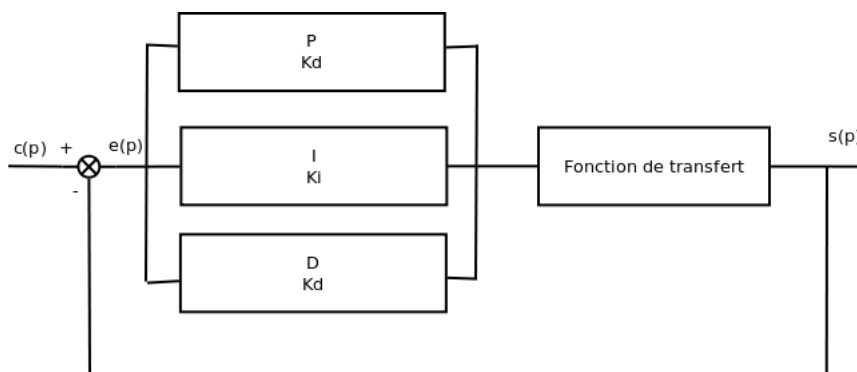
Asservissement avec régulateur PID
