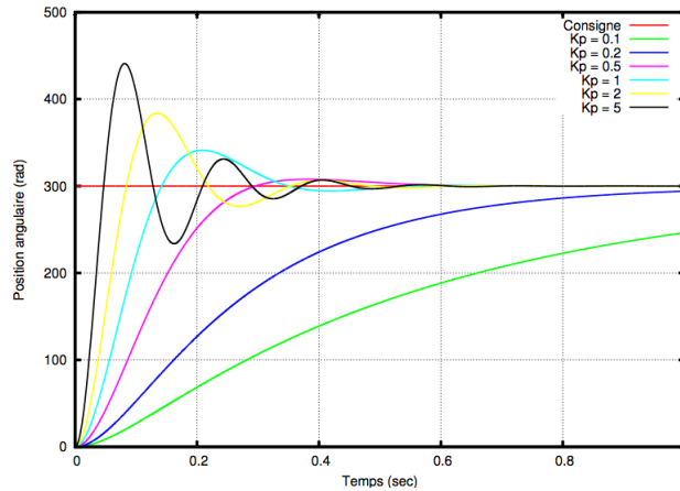
Modélisation sous Maple de la réponse à un échelon dans un asservissement en position.
