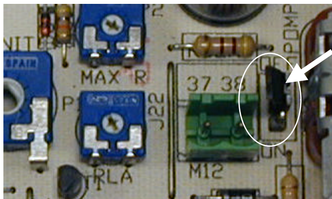
Détail de la carte montrant le shunt CM3
