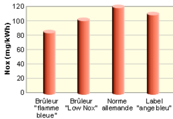
Emission de NOx des brûleurs "flamme bleue" et Low NOx comparée aux exigences des norme et label allemands
