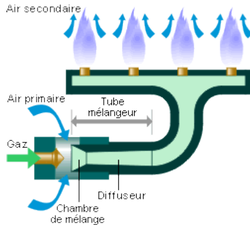
Principe de fonctionnement d'un brûleur gaz atmosphérique.
