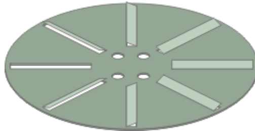
Exemple de déflecteur.
