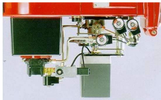
Brûleur modulant fuel
