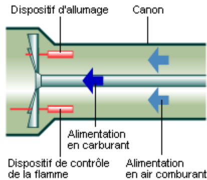
Tête de combustion d'un brûleur gaz.
