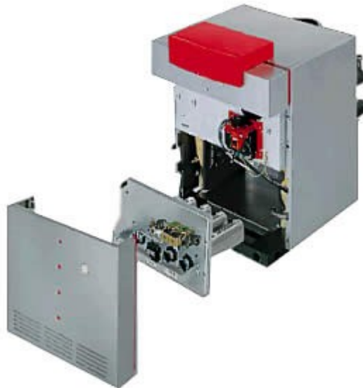
Chaudière gaz avec brûleur à prémélange total sans ventilateur.
