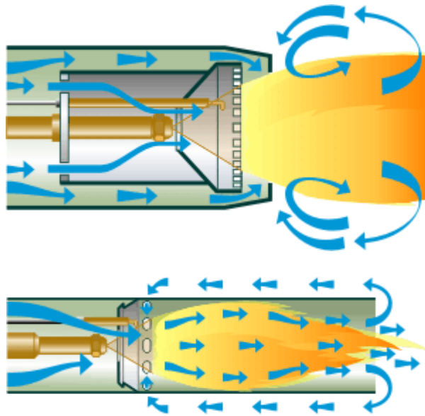
Brûleurs Low Nox.
