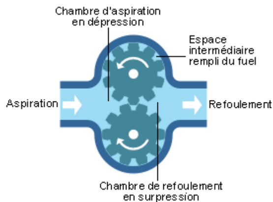
Pompe à fuel
