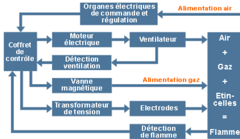
Principe de fonctionnement d'un brûleur gaz à air pulsé.
