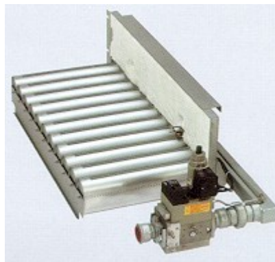
Brûleur à prémélange sans ventilateur.
