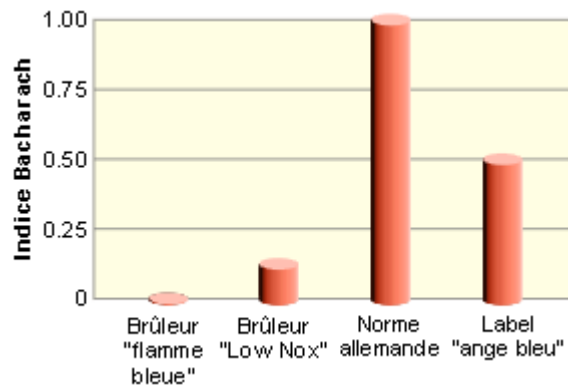
Emission de suies des brûleurs "flamme bleue" et Low NOx comparée aux exigences des norme et label allemands
