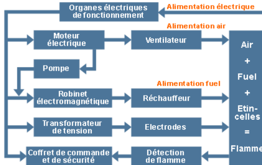
Principe de fonctionnement d'un brûleur fuel.
