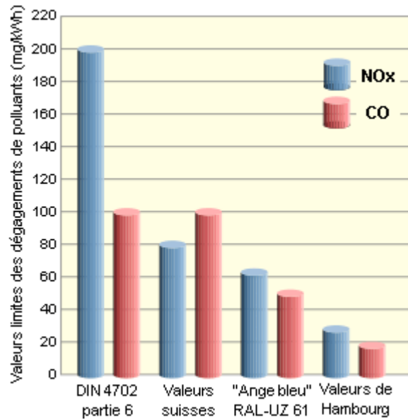
Exemples de règlements et de labels limitant la production de NO x des chaudières en Allemagne et en Suisse.
