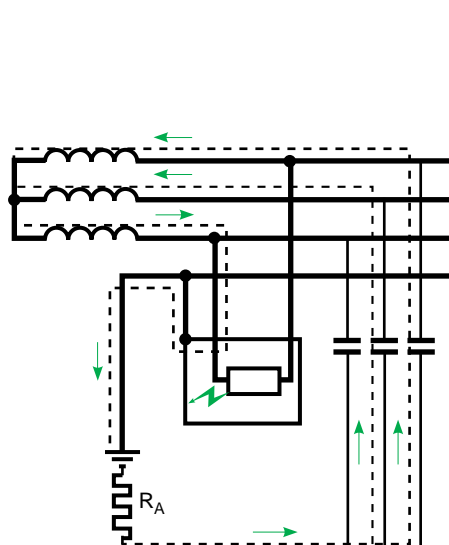
Fig. 20 : schéma IT.
