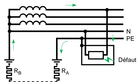
Fig. 19 : schéma TT.
