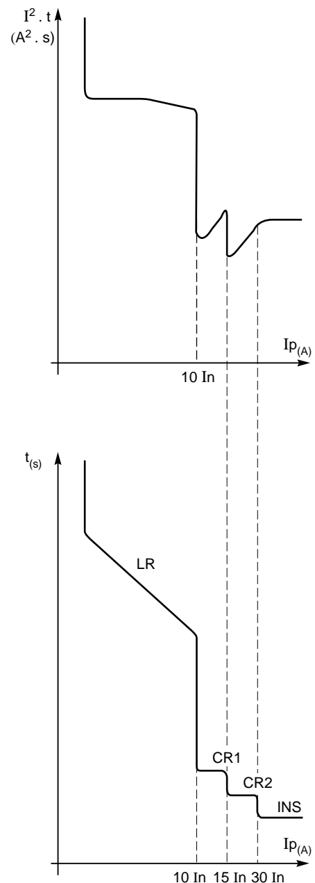
fig. 10 : courbes t_c = f(I_p) et I^2 . t = f(I_p) d'un disjoncteur équipé d'un déclencheur électronique.
