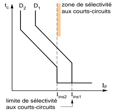
fig. 4 : sélectivité ampèremétrique.
