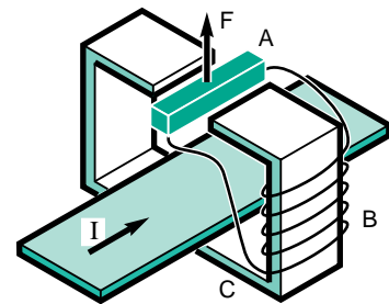
b) A circuit magnétique en C, pour disjoncteur à forte intensité nominale
