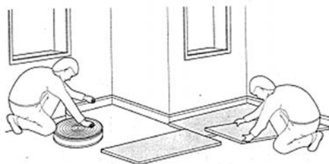
2 Pose de la bande de pourtour et de l'isolant (les joints des panneaux à bord droits doivent être recouverts d'une bande adhésive).
