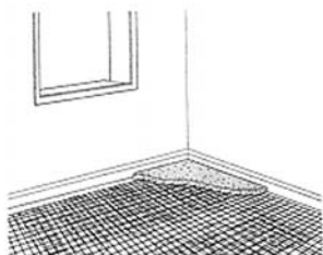
5 Pose du treillis d'armature et exécution de la chape flottante armée, avec vérification électrique des éléments après coulage.
