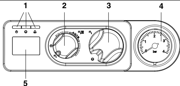
Afficheur digital (5)
