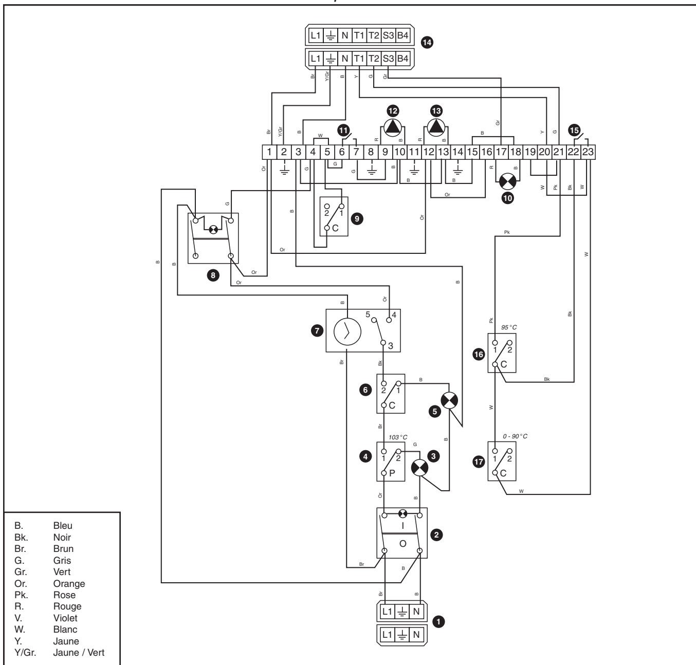
Raccordement électrique HeatMaster® 200 N / 200 F
